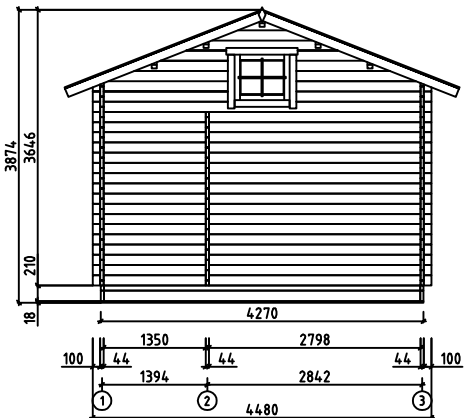
Wall- Seinä-Vägg C
