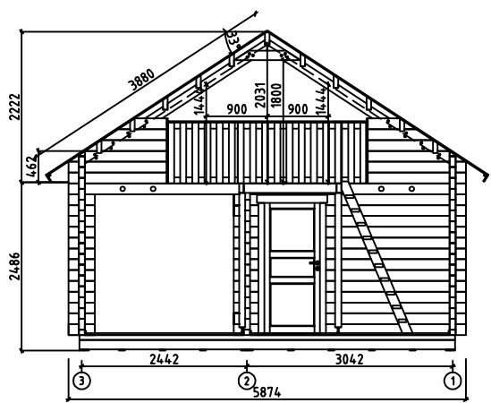
Wall- Seinä-Vägg C
