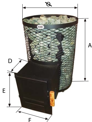
Figur 15. / Piiros 15. SY-216, SY-220
