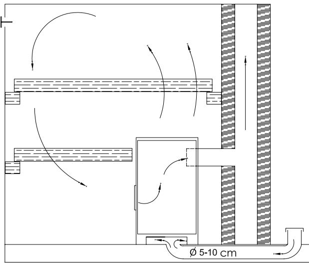
Figur 1. Naturlig ventilation Piiros 1. Luonnollinen ilmanvaihto
