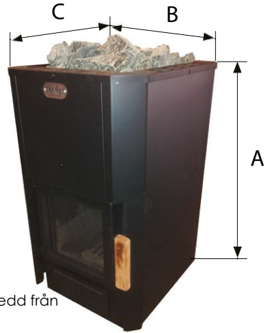
Figur 3. / Piiros 3. P-116, P-120
