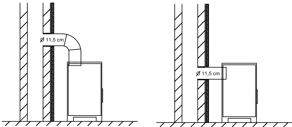
Figur 16. Anslutning av Bastuugnen till den inbyggda skorstenen. Pirros 16. Kiukaan liittäminen muurattuun savuhormiin
