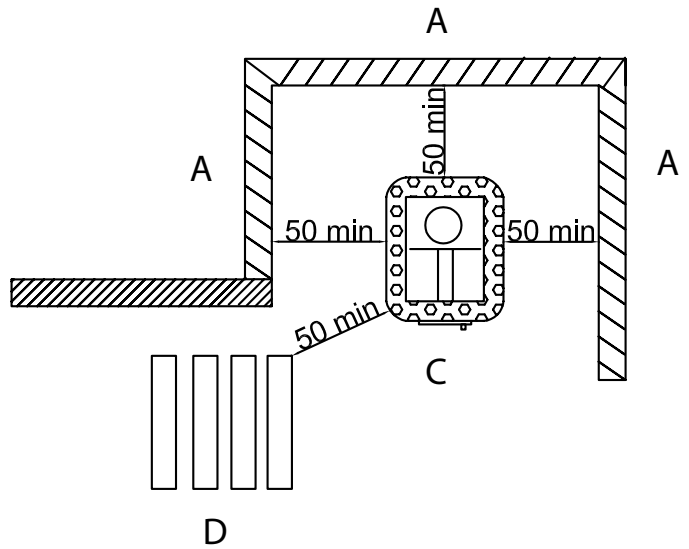
Figur 17. Säkerhetsavstånd (i cm) Piirros17 Turvavälisyydet (cm)
