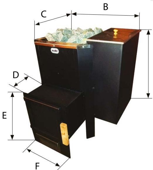
Figur 9. / Piiros 9. P-21640, P-22040
