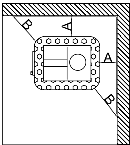
Figur 15. Säkerhetsavstånd (i cm) / Piirros15. Turvaetäisyydet (cm)
