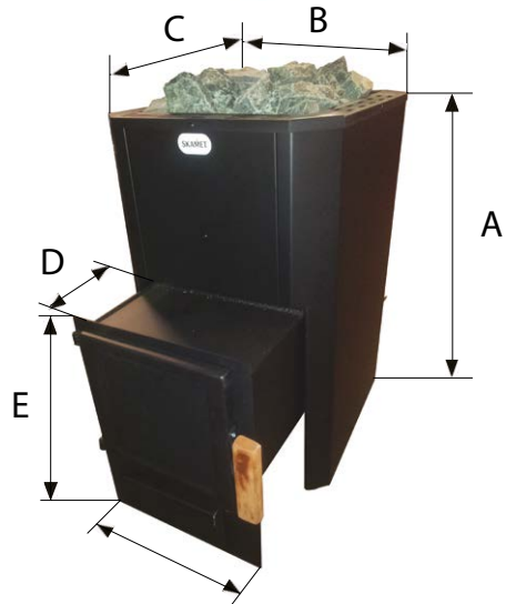
Figur 4. / Piiros 4. P-216, P-220
