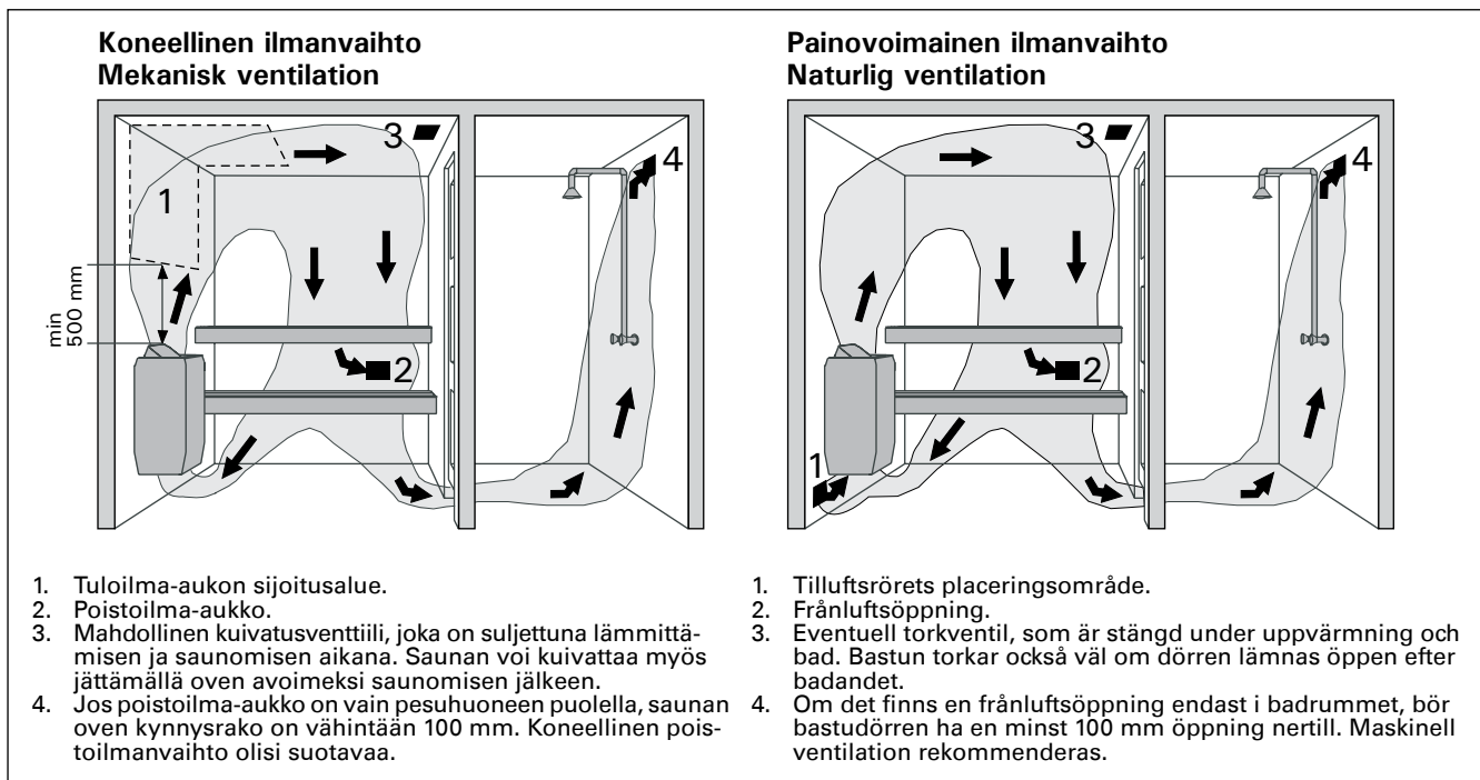
Kuva 4. Saunahuoneen ilmvaihto Bild 4. Ventilation i bastu
