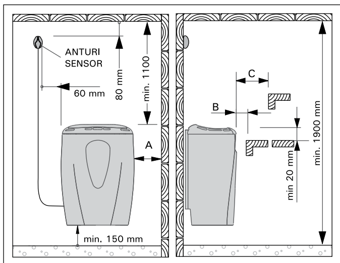
Kuva 5. Kiukaan suojeutaisydet Bild 5. Säkerhetsavstånd
