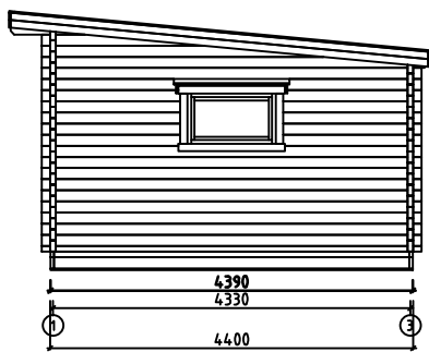
Wall- Seinä-Vägg C
