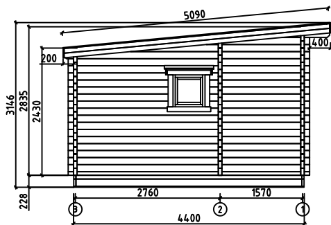
Wall- Seinä-Vägg A
