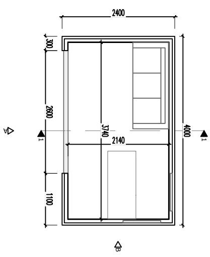
Plan 1:50
