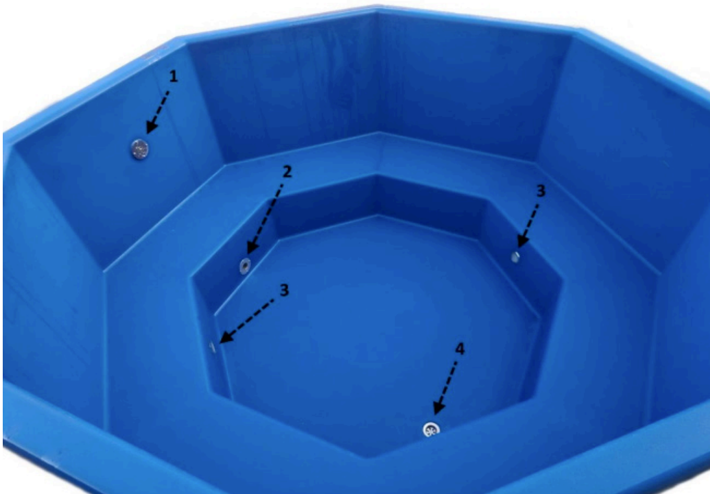
Kuva 2: Kylpytynnyrin osat
