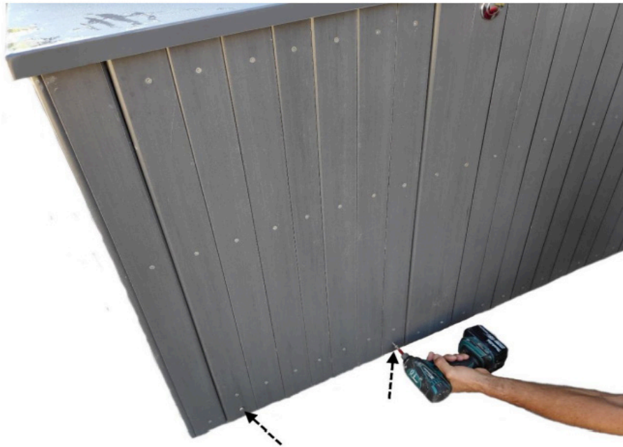
Kuva 3. Laitekaapin oven irrotus
