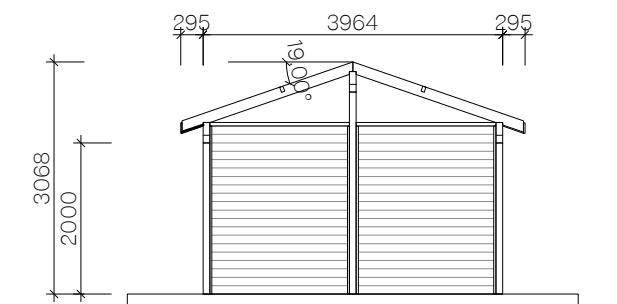
SEKTION A-A 1:100
