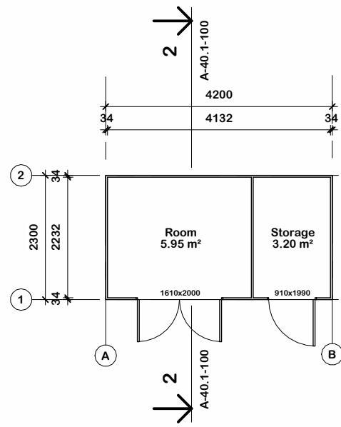
1 Plan 1 : 100
