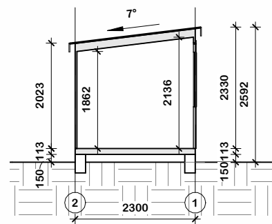
2 Section A-A 1 : 100
