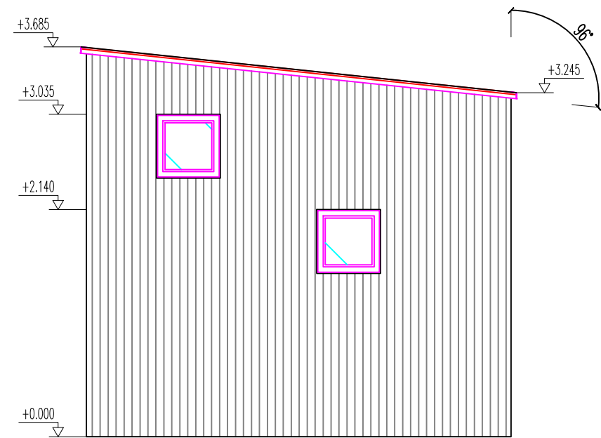
Elevation B 1:50
