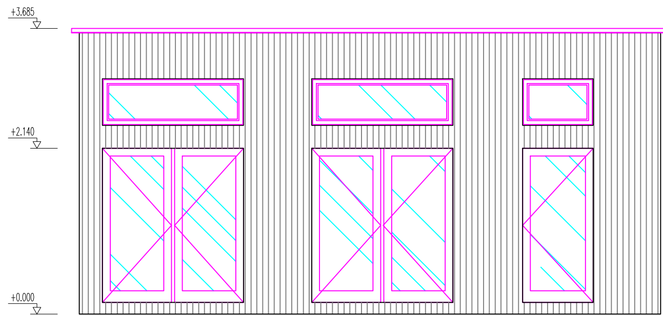
Elevation A 1:50
